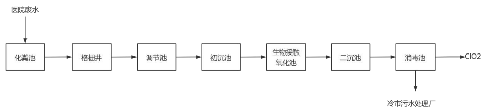
图 4-1 一体化污水处理工艺图
